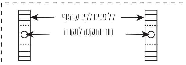
איור A - איור של גוף התאורה
